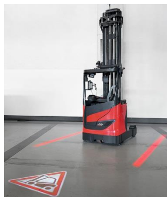
Uporaba na regalnem viličarju
